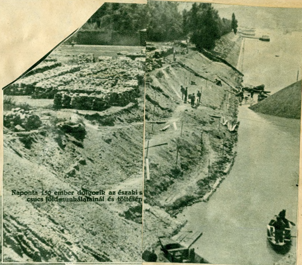
(150 méterrel meghosszabbítják a Margitsziget északi csucsát. Ide építik az óbudai híd középső főtartó pillérét. A Margitsziget meghosszabbításával megkezdődött az Árpádhíd építése, amelyet 1946-ban fejeznek be)
