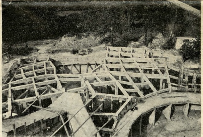
Az egyik hegyoldal lejtőjének belső cementbeton-váza s a hegyre vezető út alapozása.
