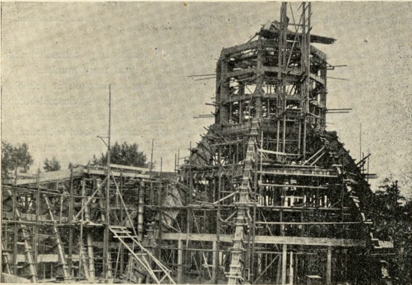
Az állatkerti nagy hegy belső váza; üres deszkatokok, melyekbe felülről a cementbetont öntik.
