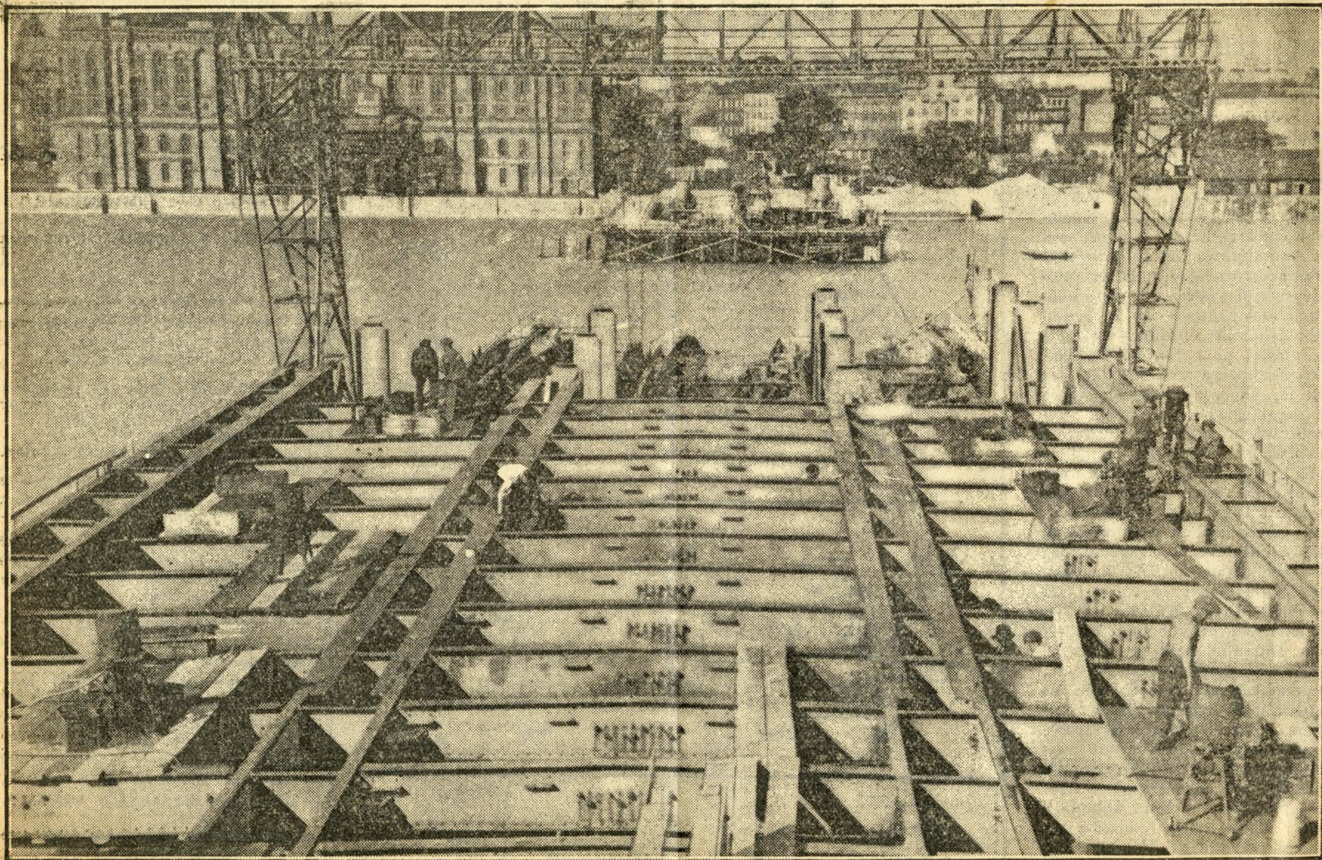
ÉPÜL A BORÁROSTÉRI HÍD. ELŐL A BUDAI OLDAL ÍVE KÉSZÜL, HATUL A PESTI OLDAL EGYIK ÍVRÉSZLETE LÁTSZIK, A KÖZÉPSŐ ÍV MUNKALATAI MÉG NEM KEZDŐDTEK MEG
