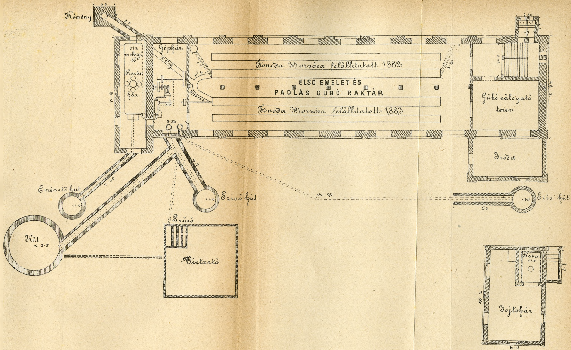
A PANCISOVAI SELYEMFONÓ GYÁR ALAPRAJZA.
