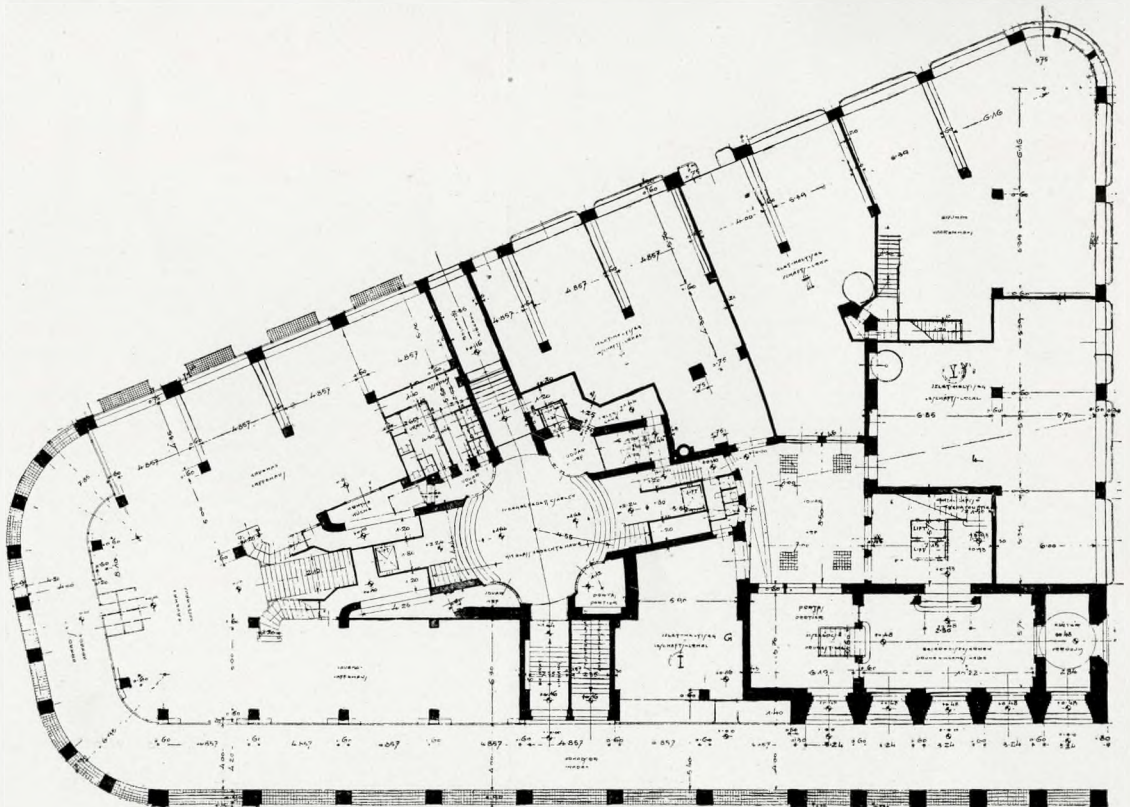
Az Adria Biztosító Társaság palotájának alaprajzai
