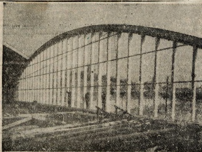
A készülő csarnok alumínium oldalváz-szerkezete
