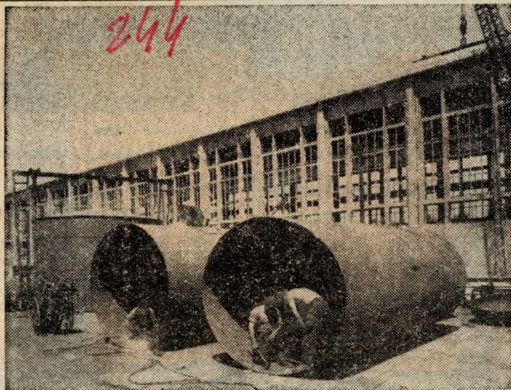
az ásványolajipar részére készülnek olajtartályok és berendezések. Ezek a tartályok a csepeli, nyírbogdányi és almásfűzitői olajfinomítóba kerülnek. Hátterben az épülő, új szerelőcsarnok.
