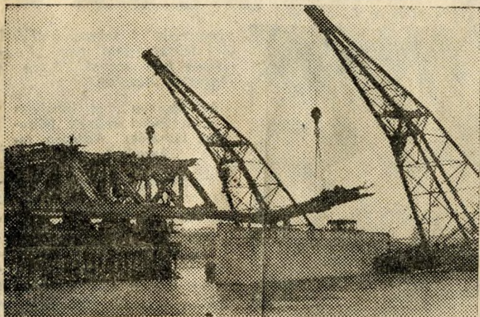
A „József Attila” és az „Ady Endre” úszódaruk beemelik a Petőfi-híd 62 tonnás alsó övtartóját.
