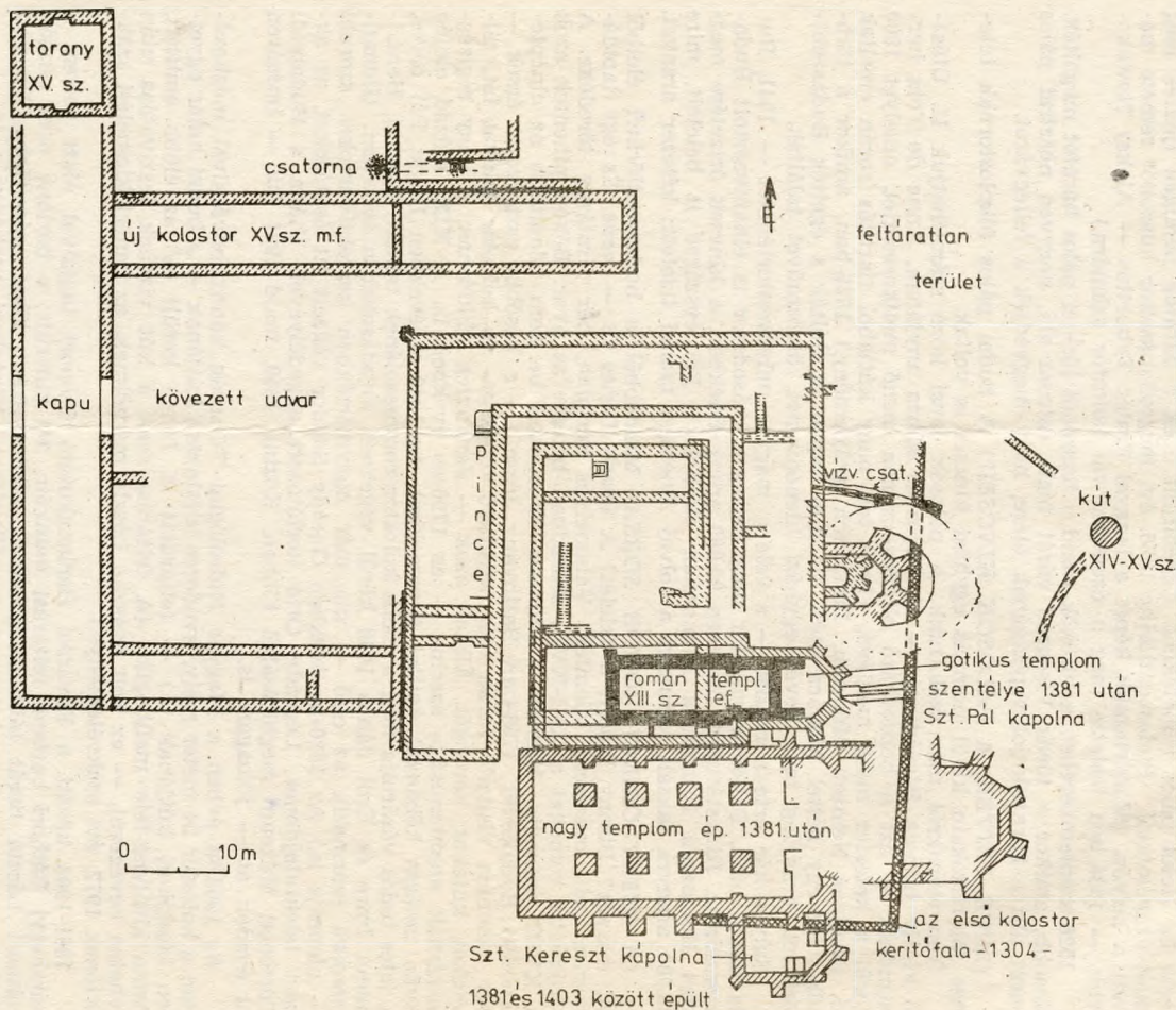
A budaszentlőrinci pálos kolostor feltárt területének alaprajza. Kuczogi Zsuzsa munkája
