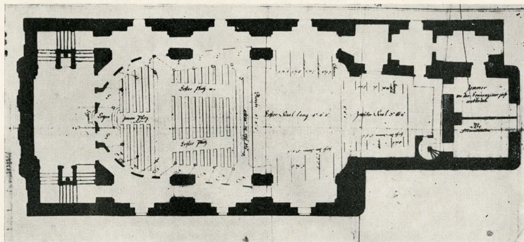
3. A színház XVIII. század végén készített alaprajza (feltehetően Kempelen Farkas terve)
