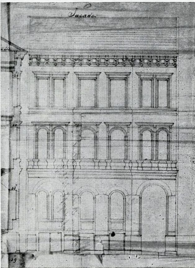
4. V. Váci u. 76. Pan József kivitelre nem került terve, 1861.
