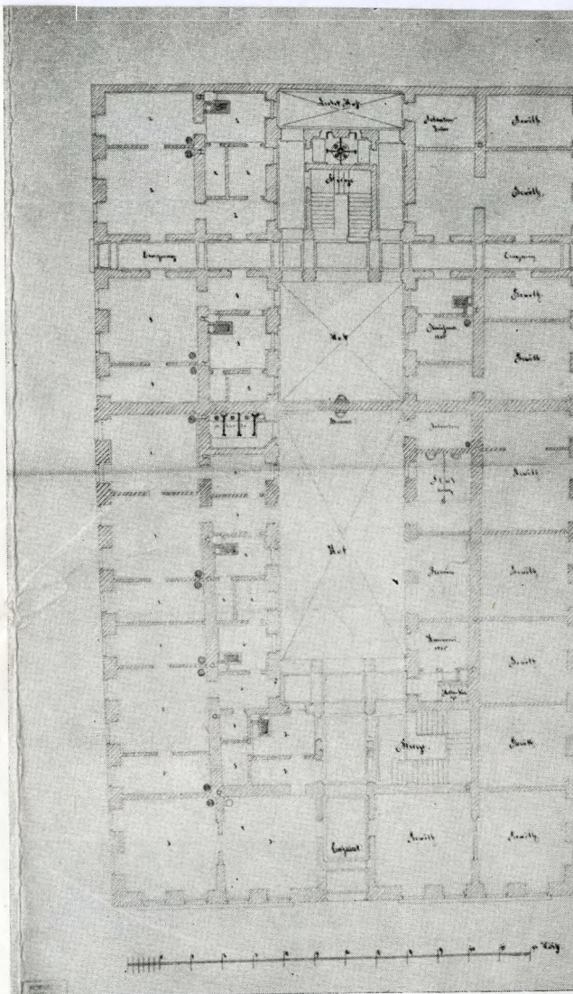
3. I. Jégverem u. 2. földszinti alaprajzának terve. Mátyásföld, 1860.
