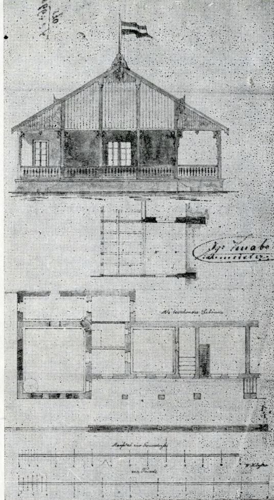
6. II. Páfrány út 17/b kiépíté- sének terve. Knabe Ignác, 1869.
