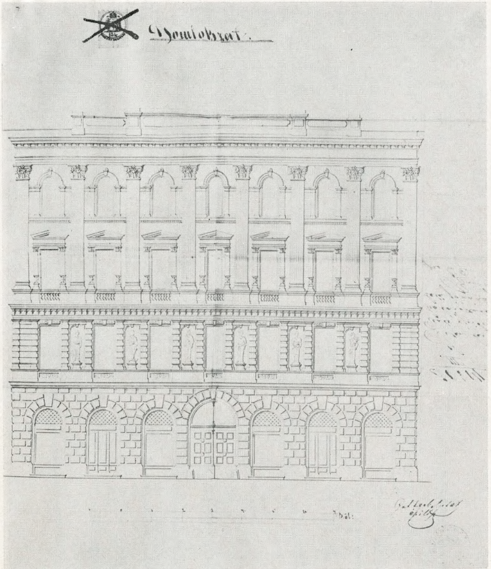
2. Budapest V., Pesti Barnabás u. 4. ház főhomlokzatának rajza
