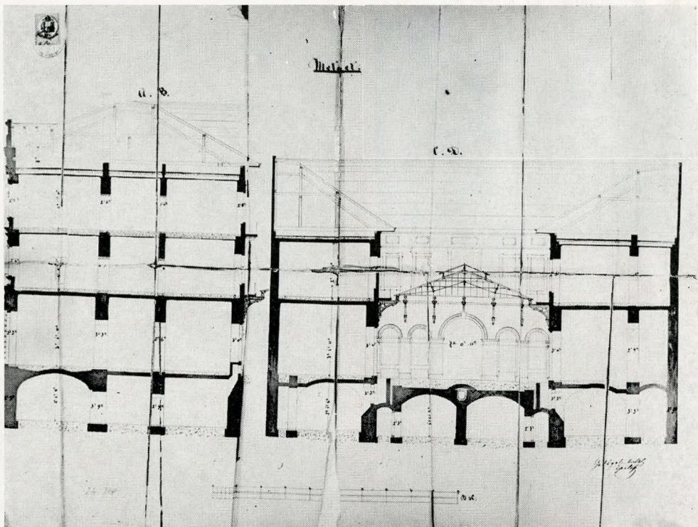
7. Az udvar lefedésének keresztmetszete
