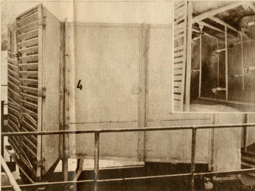
A légműködő belső és külső, szerkezeti megoldása (további képeink a következő oldalán)
