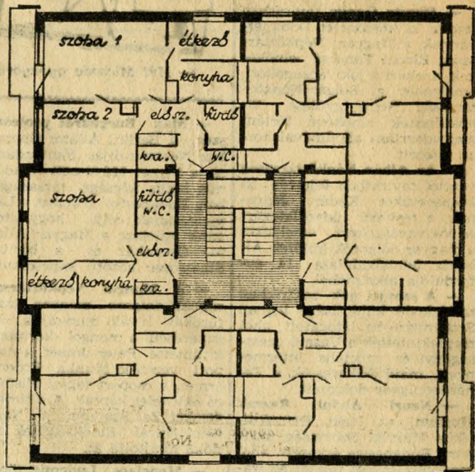
A hatlakásos kockaház emeleti alaprajzi elrendezése (Tervezők: Benjamin Károly, Boros Zoltán, Tarján László)
