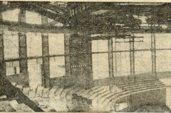
A nézőtéri lépcsőzet előregyártott vasbeton elemekből készült. A fordított U-alakú elemek fogazott vasbeton gerendákra ülnek
