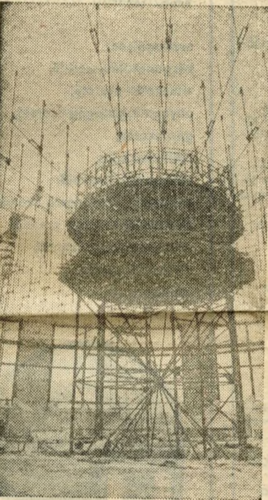
A szovjet acélszerkezet építése a húzott gyűrűket alátámasztó állványtorony megépítésével kezdődött
