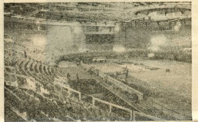
A belső csarnoktérben több szakipari munka egyszerre készült: a világítási és hangosítási rendszer szerelése, az eredményhirdető próbáuzemelés, a nézőtéri ülések elhelyezése
