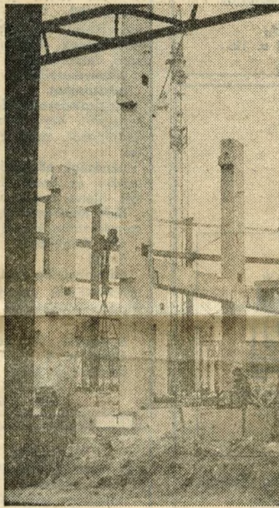
A kábeltetőt tartó 48 acéloszlop vasbeton alaptesteken áll
