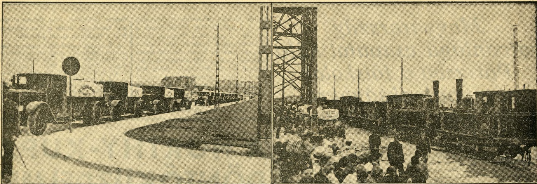
VIZZEL TELT LOCSOLÓAUTÓK, MOZDONYOK ÉS MEGTERHELT VASÚTI KOCSIK DÜBÖRÖGTEK VÉGIG AZ ÚJ HIDON, AMELY KITŰNŐEN BIRTA A TEHERPRÓBÁT
