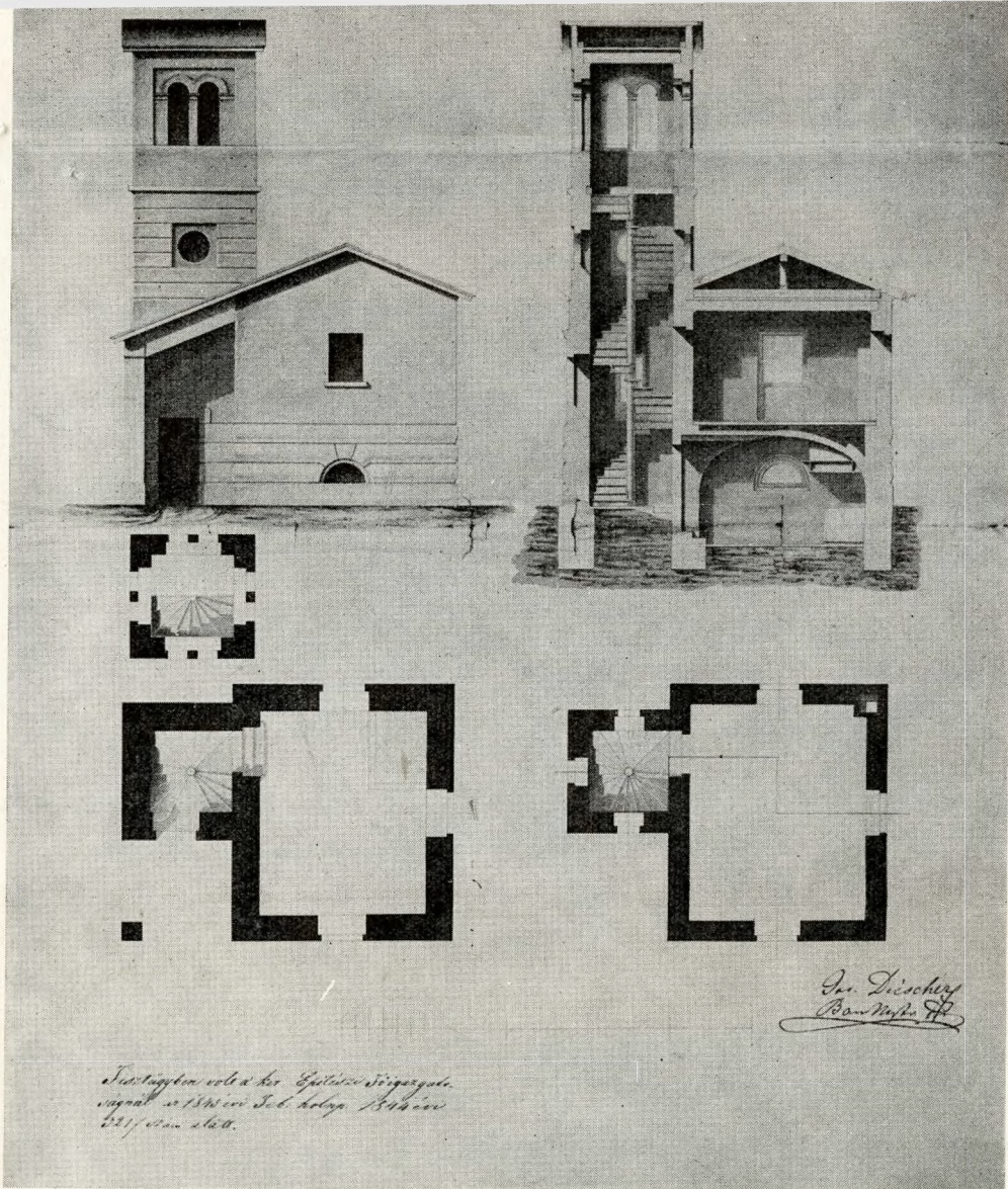
6. A kőbánya csőztorony terve (nem valósult meg)
