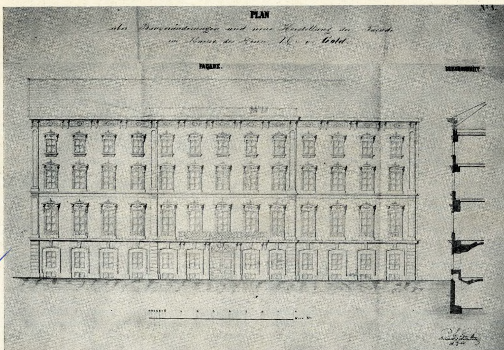
5. VI., Paulay Ede u. 33. ház részben kivitelezett terve (Pollack Mihály, 1833)
