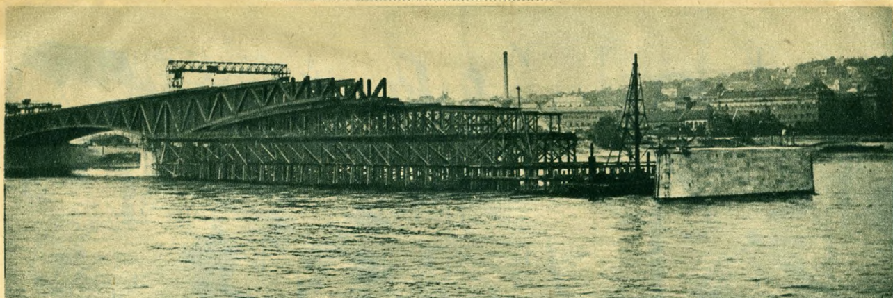
Az épülő Boráros-terti híd; a híd vasszerkezetének több mint a fele már megépült.
