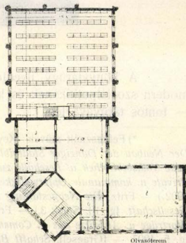
3. ábra: A danzigi városi könyvtár alaprajza. (Mértéke 1:600. — 1 cm = 6 méter.)
