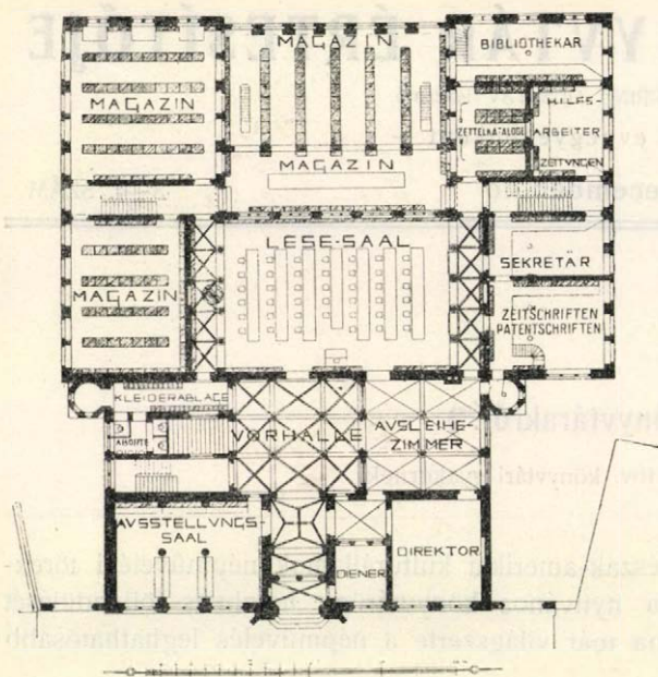
2. ábra: A kőlni városi könyvtár alaprajza. (Mértéke 1:600. — 1 centiméter = 6 méter.)
